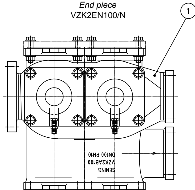
Zwischenstück mit Abgabeanschluß Intermediate piece with connector VZK2AB100/N
