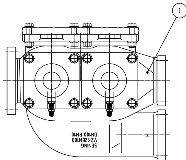
Endstück End piece VZK2EN100/N
