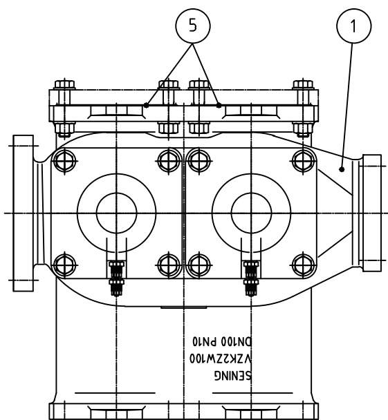
Zwischenstück ohne Abgabeanschluß Intermediate piece without connector VZK2ZW100/N
