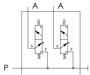
Schaltbild Connection scheme
